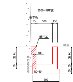
2号水路工
