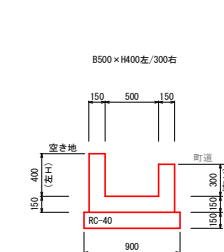
3号水路工
