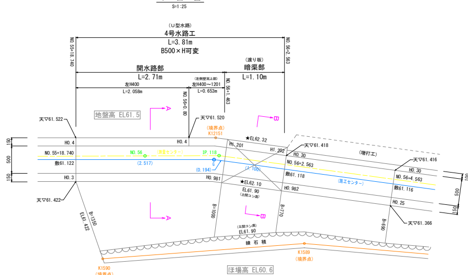
平面图
