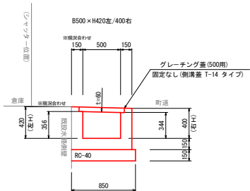
2号水路工
