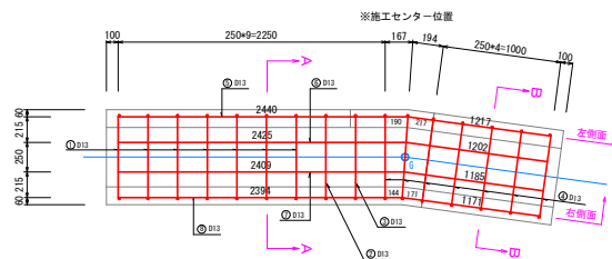
配筋図 S=1:25
