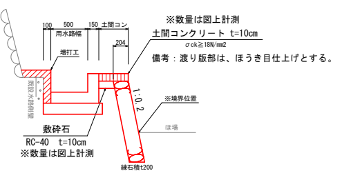
土間コンクリート S=1/25
