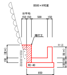
3号水路工
