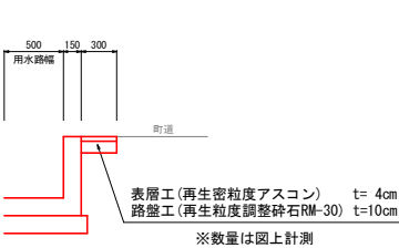
舗装構成(AS舗装復旧) S=1/25
