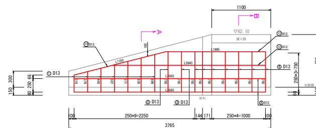
(右側面)
