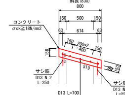
渡り版工
