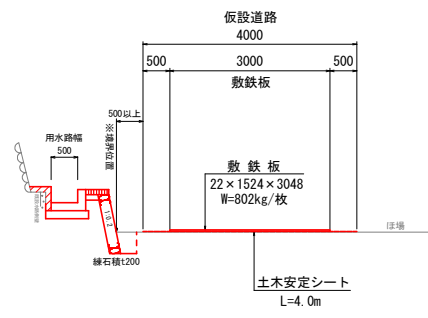
仮設道路・標準図 S=1:50
