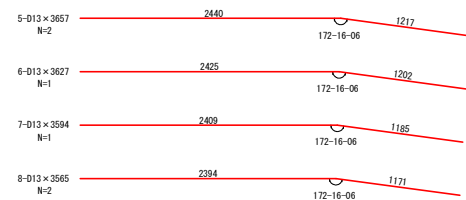
配筋図 S=1:25
