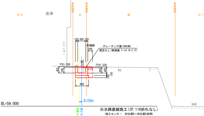
水路断面 B500×H420(左)/400(右)・・・側壁外高(グレーチング蓋付)
