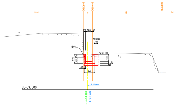
水路断面 B500×H541
