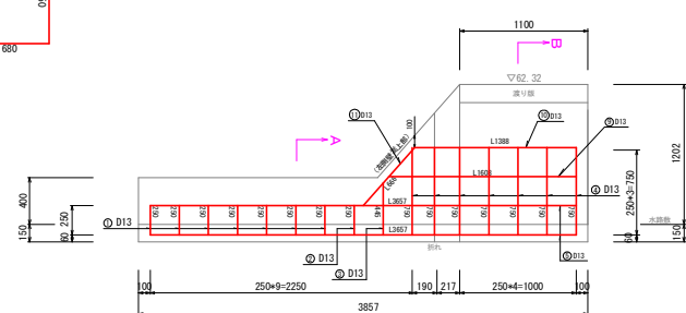
(左側面)
