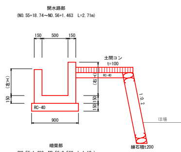
4号水路工
